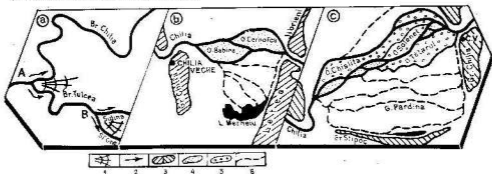
Fig. 4. Tipuri de difluențe :
