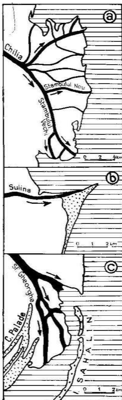
Fig. 9. Microdeltele de la gurile celor trei brațe :
