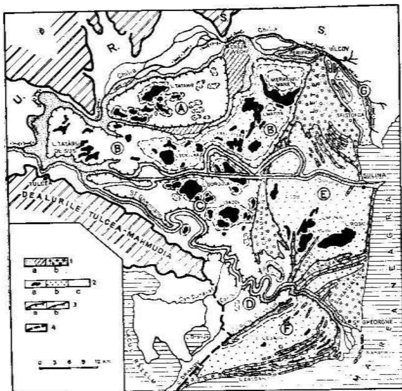
Fig. 7. Marile zone depresionare ale deltei cu grindurile și cordoanele marginale : 1 — relieful pozitiv : a — grinduri fluviale (cu hașură oblică grinduri continentale) ; b — cordoane marine ; 2 — relieful negativ — depresiuni deltaice : a — lacuri principale ; b — porțiuni sub 0 m marin (după C. Brătescu) ; c — restul depresiunilor ; 3 — limitele depresiunilor deltaice ; a — în delta fluvială ; b — în delta fluvio-maritimă ; 4 — limita de sud-vest a deltei. A — depresiunea Pardinei ; B — depresiunea Sireasa—Fortuna—Matîța ; C — depresiunea Gorgovei ; D — depresiunea Erenciuc—Cerneț ; E — depresiunea Sulinei ; F — depresiunile Lejaiu—Zătoane ; G — depresiunea Sfiștofca—Vilcov.
