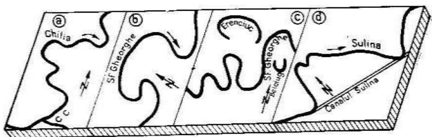
Fig. 6. Tipuri de meandre :
