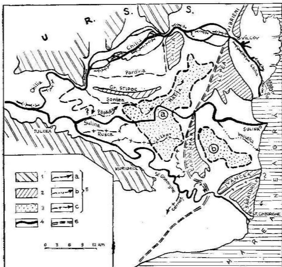
Fig. 5. Sistemele de brațe principale și secundare și formarea lor prin procesul de difuziune :
