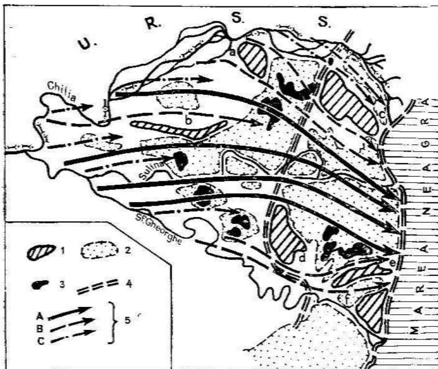
Fig. 15. Procesul de inundabilitate :
