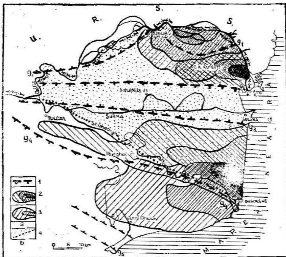
Fig. 2. Schița structurilor geologice de tip bloc ale fundamentului hercincico-chimeric al deltei;
