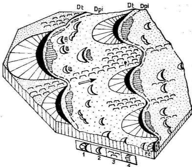
Fig. 13. Un exemplu de dune transversale și longitudinale mobile din zona de acumulare internă (Dt — dune transversale; Dpi — depresii interdunare): 1 — barcane mari; 2 — barcane mici; 3 — dune longitudinale; 4 — porțiunile cele mai adânci din fruntea dunei mari de tip barcană.
