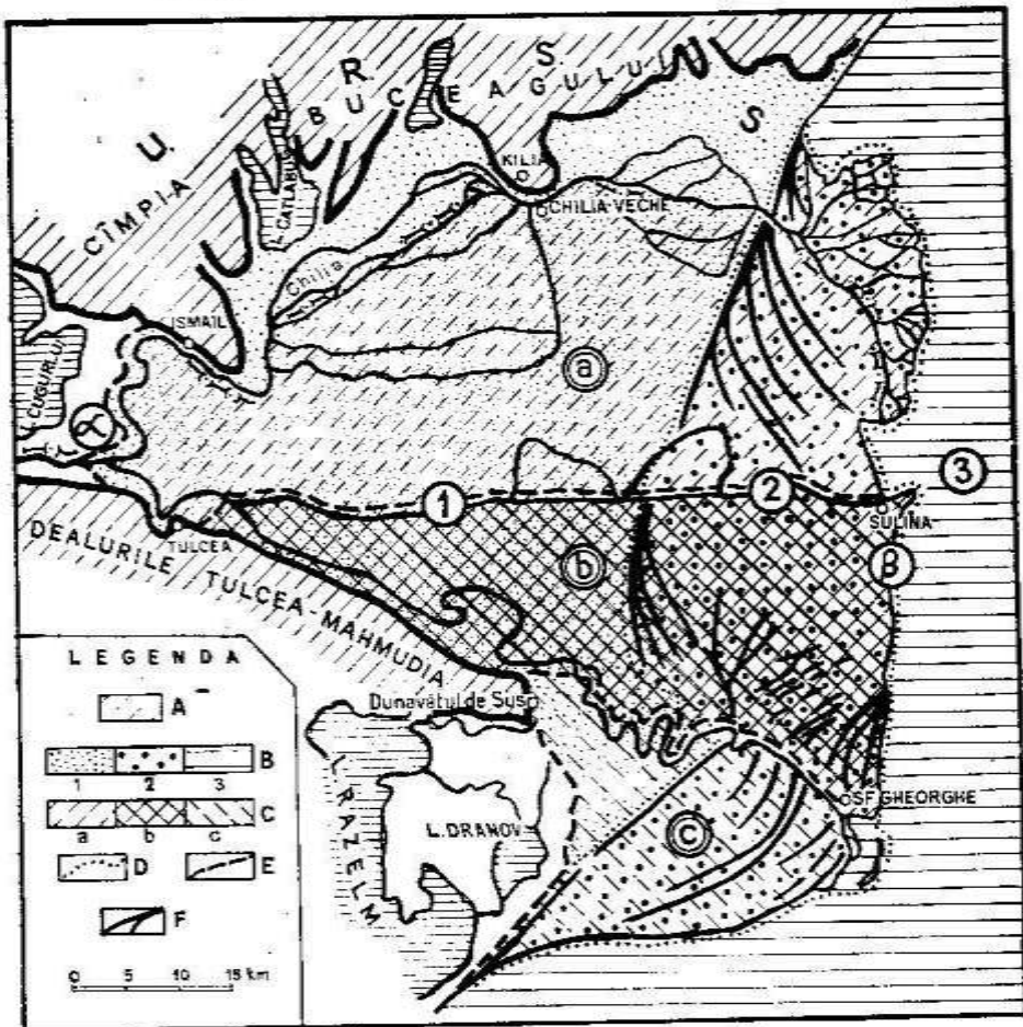
Fig. 1. Marile compartimente ale Deltei Dunării; A — Cadrul învecinat înalt. B — Subdiviziunile transversale: 1-deltă barată (fluviațilă sau fluvio-limnică); 2-deltă liberă (fluvio-maritimă); 3-predelta (zona litorală predeltaică). C — Subdiviziunile longitudinale — macroostrovele: a-ostrovul dintre brațele Chilia și Tulcea—Sulina (nordic); b-ostrovul dintre brațele Sulina și Sf. Gheorghe (central); c-ostrovul dintre brațul Sf. Gheorghe—Dunavăț și Dranov (sudic). D — Limite transversale. E — Limite longitudinale. F — Direcția cordoanelor principale. \alpha — vârful deltei; \beta — baza deltei.
