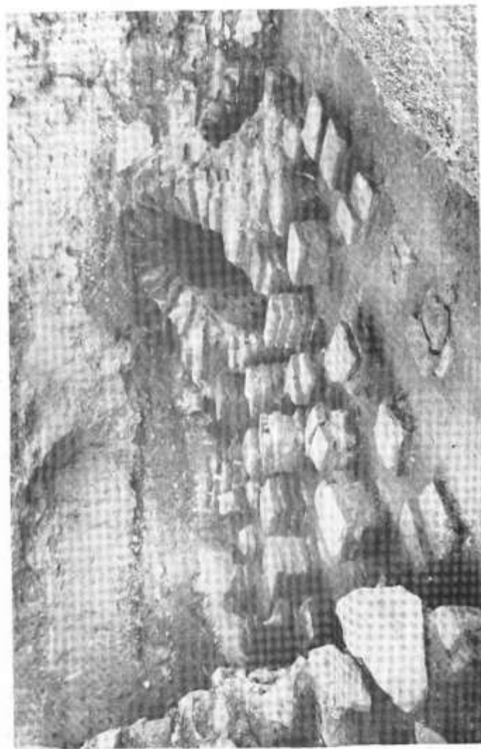
Pl. III — Noviodunum : hypocaustul unor terme romane.
