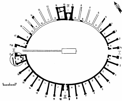
Fig. 1. Porolissum, amfiteatrul de piatră. (după Bajusz 2003b).
